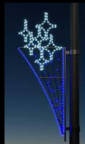
RL-FD-040* 51x137cm 220 B 24 Вт IP 65
